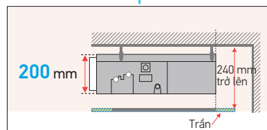
Hình chiếu cạnh
