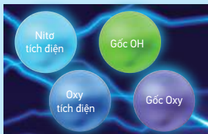
Các electron va chạm và kết hợp với nitơ và oxy trong không khí để tạo thành bốn loại nguyên tử bất hoạt với sức mạnh bất hoạt.
