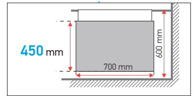
Hình chiếu bằng
