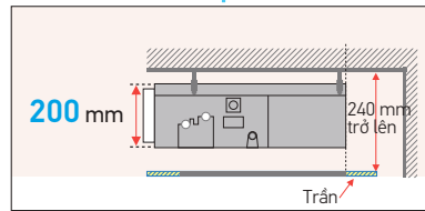
Hình chiếu cạnh
