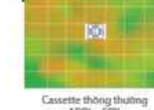
Cassette thông thường ADPI ~ 68%
